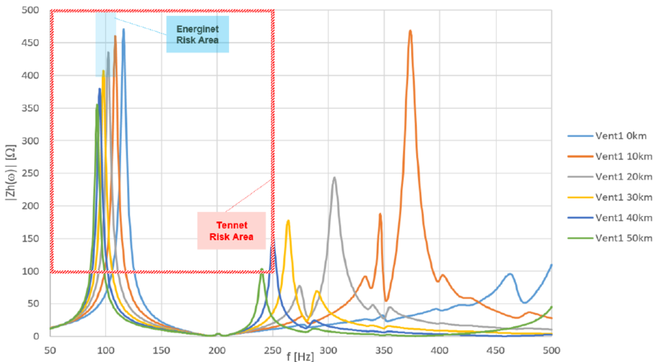
Figuur 33 - Resonantiespectra van de Ventilus corridor, voor verschillende kabellengtes, met aanduiding van de gevaarlijke zones volgens Energinet (blauwe zone) en Tennet (rood omlijnde zone).
